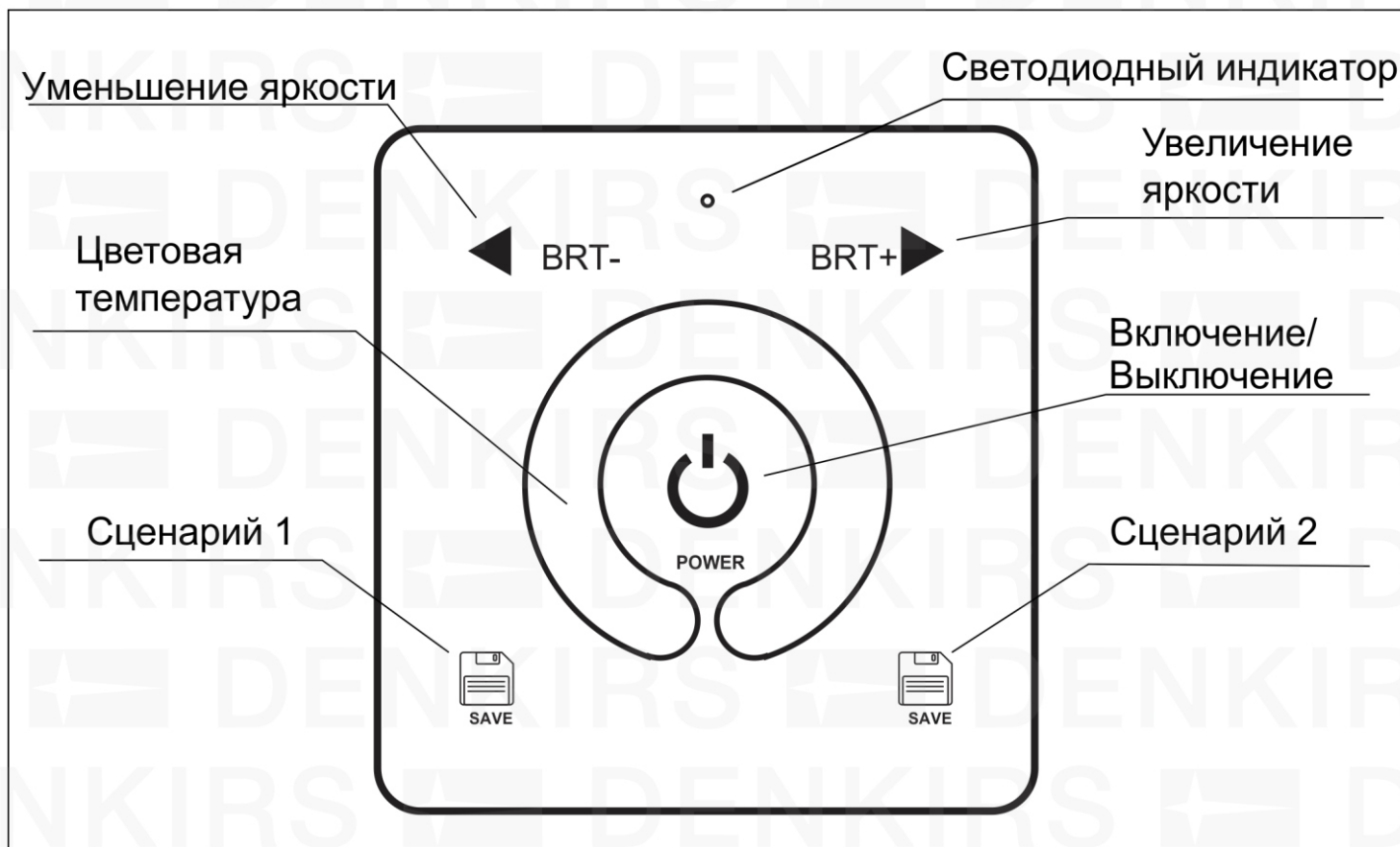
Рис. №3. Кнопки регулировки на сенсорной панели.
