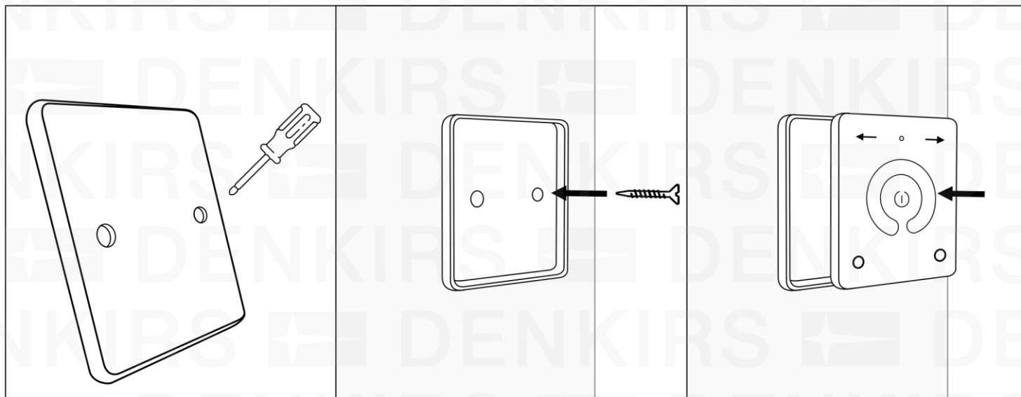
Рис. №2. Схема установки панели на саморезы
